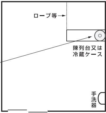
(図C) 管理建築物内で弁当等を 一時的に販売する場合
